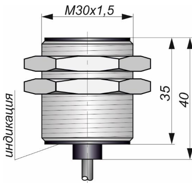
Габаритный чертеж
